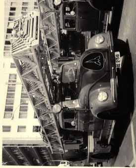
Κλιμακοφόρο 50 μέτρων Magirus Deutz Jupiter, προμήθειας 1960.
