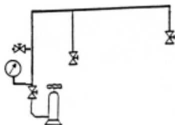
Εικόνα 10.2 Δοκιμή στεγανότητας
