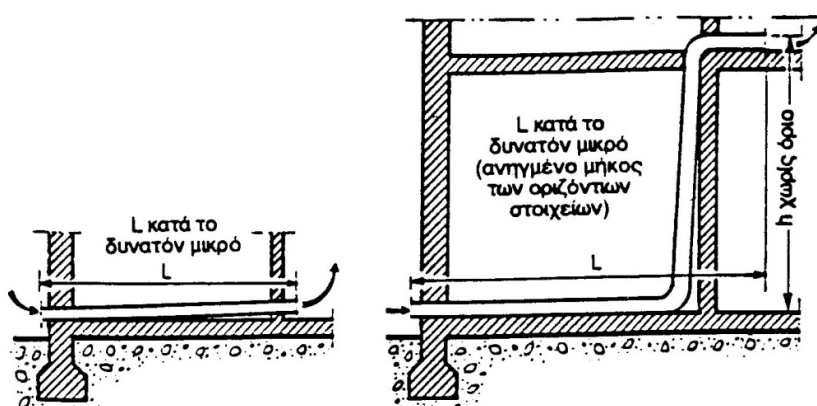
Εικόνα 8.4 Παραδείγματα οδήγησης αγωγών τροφοδοσίας αέρα
