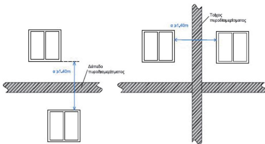
Σχήμα 26: Απόσταση ανοιγμάτων σε εξωτερικές τοιχοποιίες
