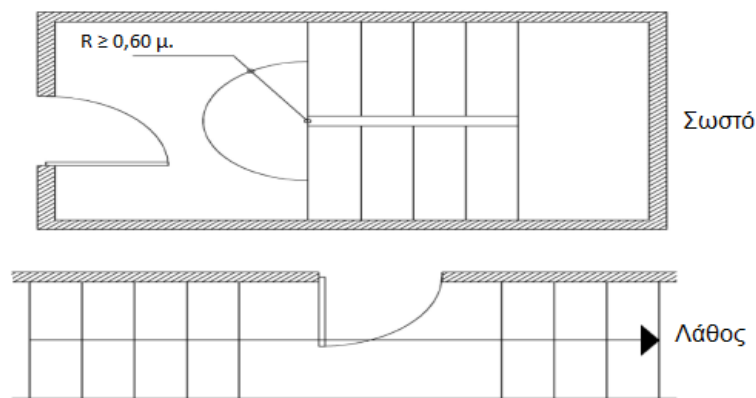
Σχήμα 4 Θύρες κλιμακοστασίων
