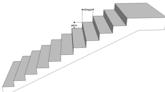
Σχήμα 6 Βαθμίδες κλιμάκων
