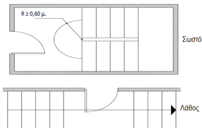
Σχήμα 5 Θύρες κλιμακοστασίων
